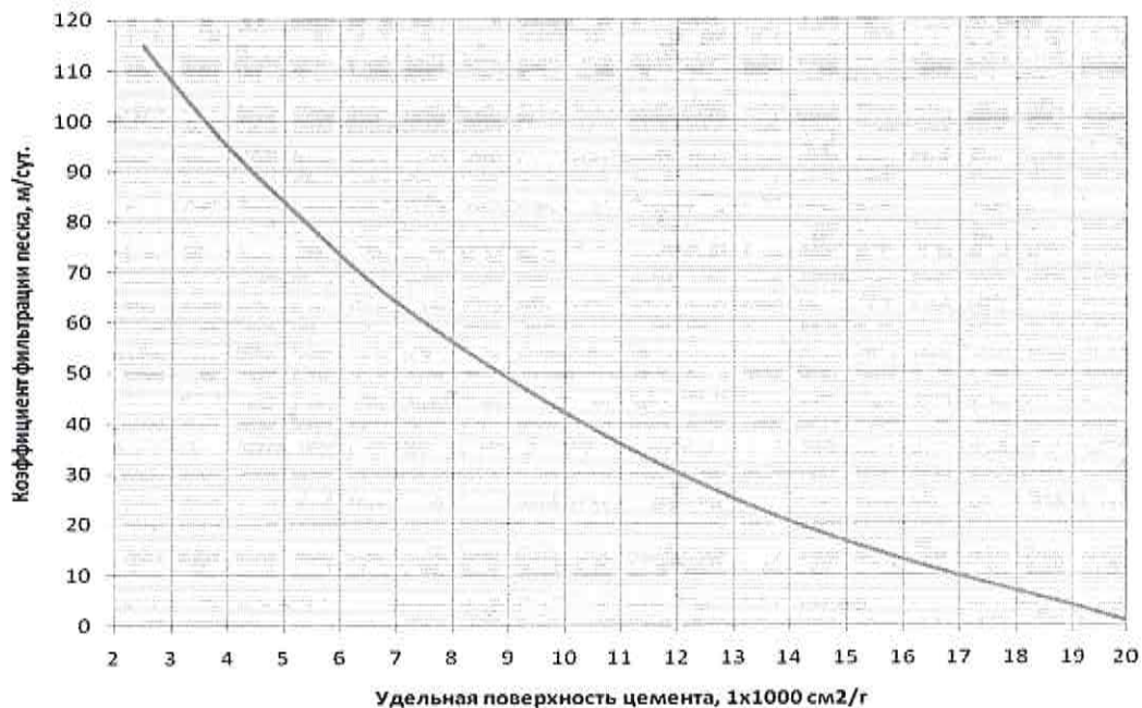
Рисунок Т.1 – График зависимости проникающей способности цементного раствора от удельной поверхности цемента и K_f
