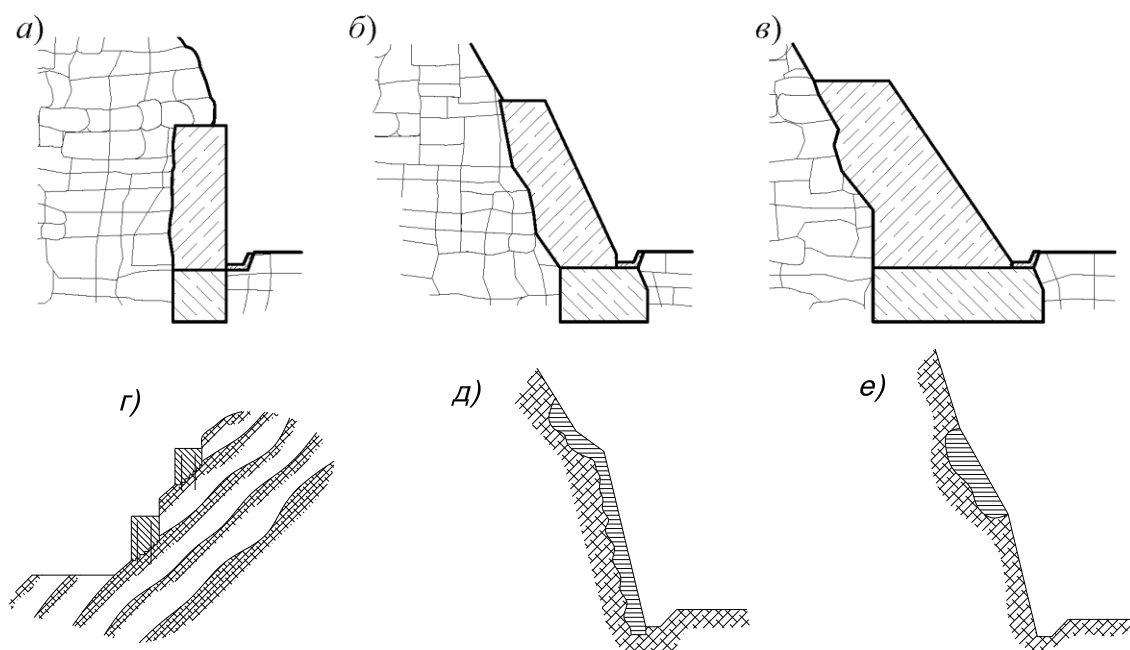
a – поддерживающая стена; б – подпорная стена; в – контрфорс; г – опояски; д – облицовочная стена; е – пломба
