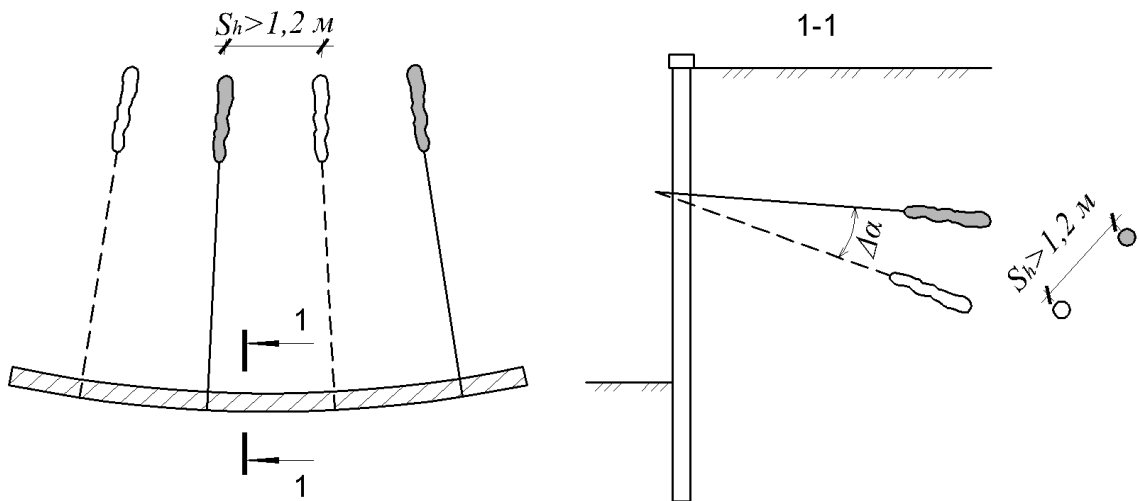
Рисунок 6.10 – Расположение анкеров на криволинейных участках сооружения
