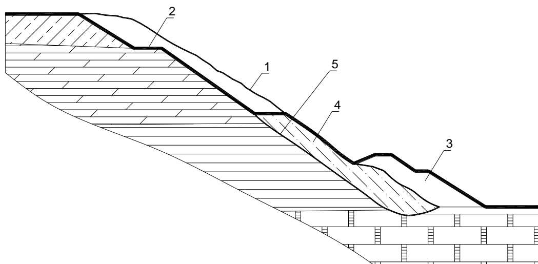
1 – поверхность исходного склона; 2 – поверхность террасированного склона; 3 – контрбанкет; 4 – оползневой массив; 5 – вероятная поверхность скольжения оползневого массива
