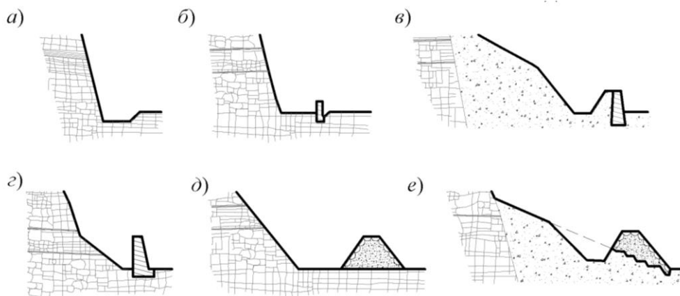
a – улавливающая траншея; b – улавливающая полка с бордюром; в – улавливающая стена; г – оградительная улавливающая стена; д – улавливающий вал у подошвы; е – улавливающий вал на склоне
