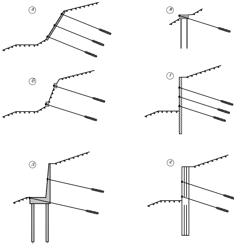
a – с опорной плитой; б – с поясами в виде балок; в – в составе однорядного или многорядного ростверка; г – для крепления подпорной стены; д – для крепления подпорной стены на свайном фундаменте; е – для крепления столбчатой (контрфорсной) конструкции
