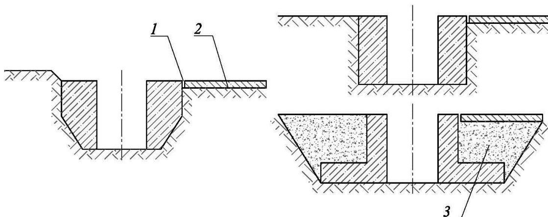
1 – деформационный шов; 2 – технологическая дорога; 3 – обратная засыпка
