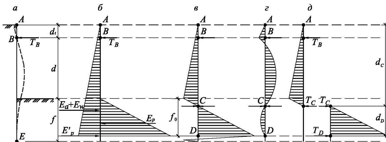
a – деформированная схема конструкции; б, в – последовательная аппроксимация активного и пассивного давления; z – эпюра изгибающих моментов в стене; д – разбиение конструкции на эквивалентные балки; d_t – глубина установки яруса крепления; d_c – глубина точки нулевого момента в стене; C – точка нулевого момента в стене; T_B – усилие в элементе крепления; T_C и T_D – усилия в условных опорах; d_D – расстояние от точки C до точки D
