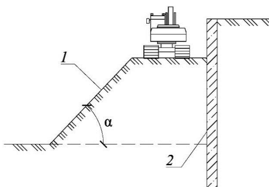
1 – грунтовая берма; 2 – подпорное сооружение; α – угол откоса бермы (определяется по расчету)
