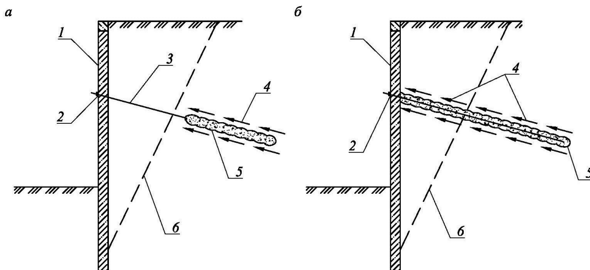
a – со свободной длиной; б – без свободной длины; 1 – подпорное сооружение; 2 – оголовок анкера; 3 – тяга анкера (свободная длина); 4 – трение по грунту; 5 – корень анкера (цементное тело); 6 – теоретическая граница призмы активного давления
