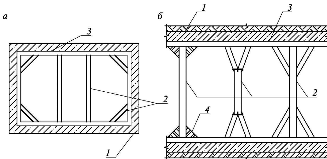
а – схема расстановки распорных элементов в плане при рядовом шаге распорок; б – примеры узлов опирания распорных элементов при большом шаге распорок в плане; 1 – подпорное сооружение; 2 – распорка; 3 – распределительный пояс; 4 – лист
