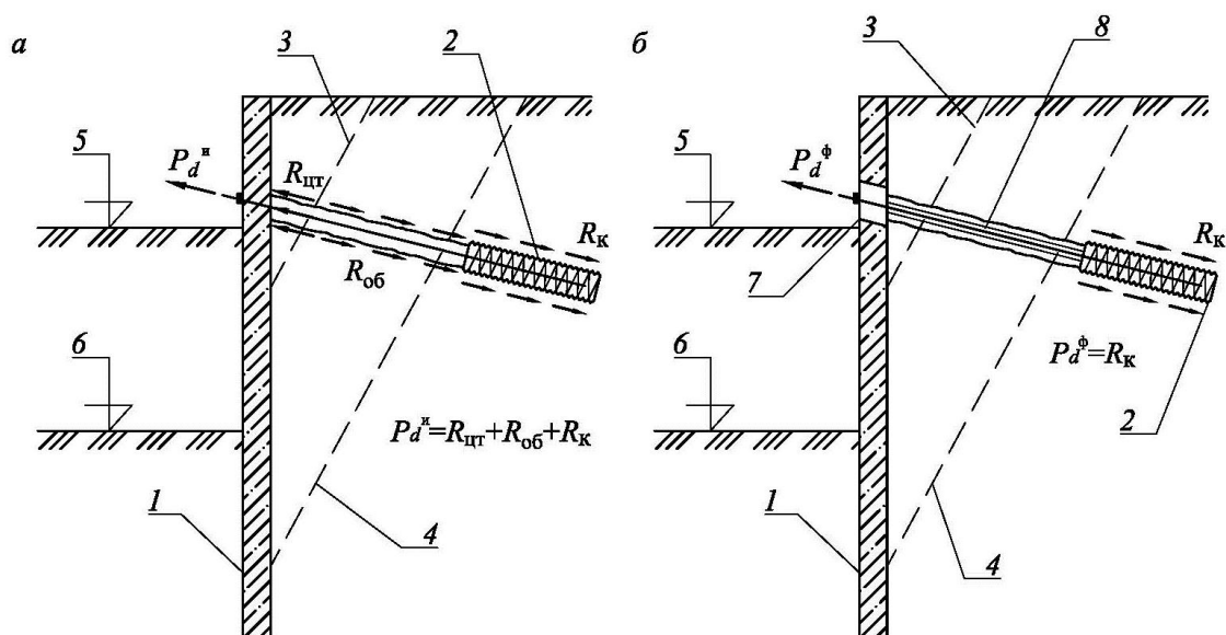
Рисунок 8.11 – Винтовая штанга
