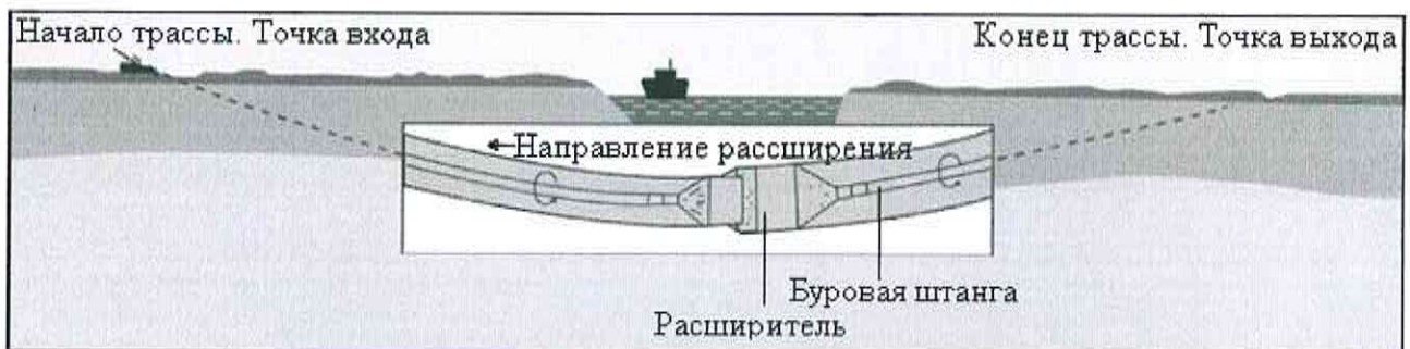
Рисунок 8.4 – Расширение скважины
