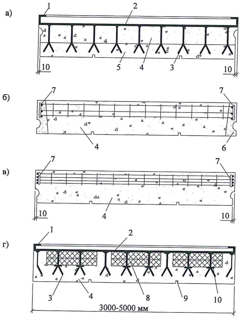
а – двухслойная панель на металлическом листе; б – панель с окаймляющим каркасом из тяжелого жаростойкого бетона; в – панель с окаймляющим арматурным каркасом; г – панель на металлическом листе со стальными анкерами и эффективной теплоизоляцией; 1 – уголок жесткости панели; 2 – металлический лист; 3 – анкер; 4 – легкий жаростойкий бетон с D1100 и менее; 5 – легкий жаростойкий бетон с D1200 и более; 6 – окаймляющий каркас из тяжелого жаростойкого бетона; 7 – арматурный каркас; 8 – эффективная теплоизоляция; 9 – усадочный шов; 10 – шайба
