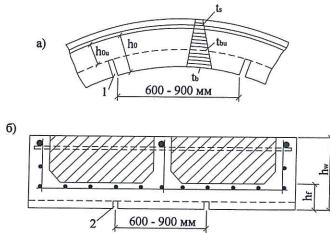
a – компенсационные; b – усадочные; 1 – компенсационный шов шириной 2–5 мм; 2 – усадочный шов глубиной 0,1h_f и шириной 2–3 мм
