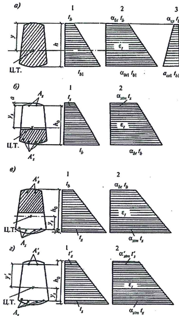
a – бетонного и железобетонного элемента без трещин; b – железобетонного элемента с трещинами в растянутой зоне, расположенными у менее нагретой грани; в – то же, у более нагретой грани; г – железобетонного элемента с трещинами по всей высоте сечения; Ц.Т. – центр тяжести приведенного сечения
