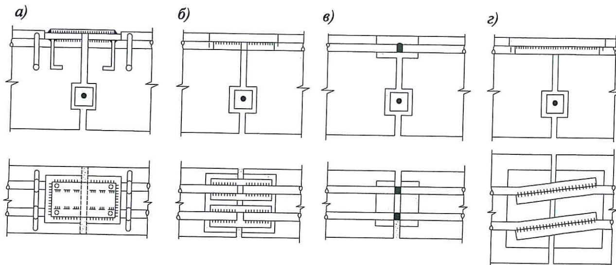
a – нахлесточное соединение с металлической накладкой из листовой стали; б – стыковое соединение по ГОСТ 10222; в – стыковое соединение по ГОСТ 14098; г – нахлесточное соединение
