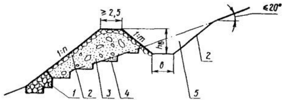
Рис. 38. Схема устройства улавливающего рва на косогоре крутизной до 20^\circ :
