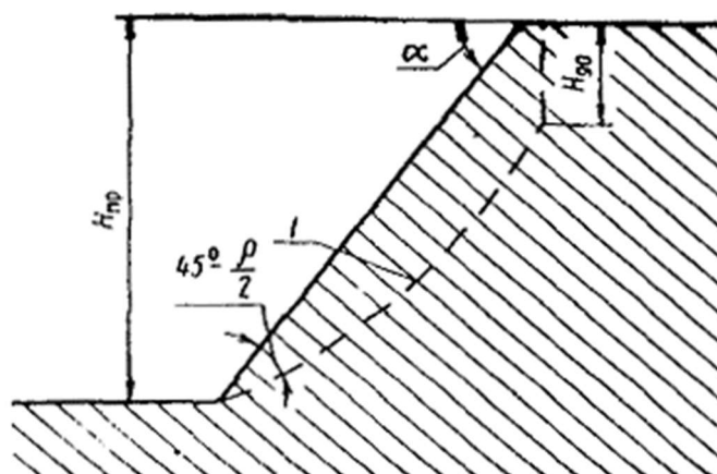
Рис. 4. Расчетная схема наклонного откоса при благоприятном расположении плоскостей ослабления:
