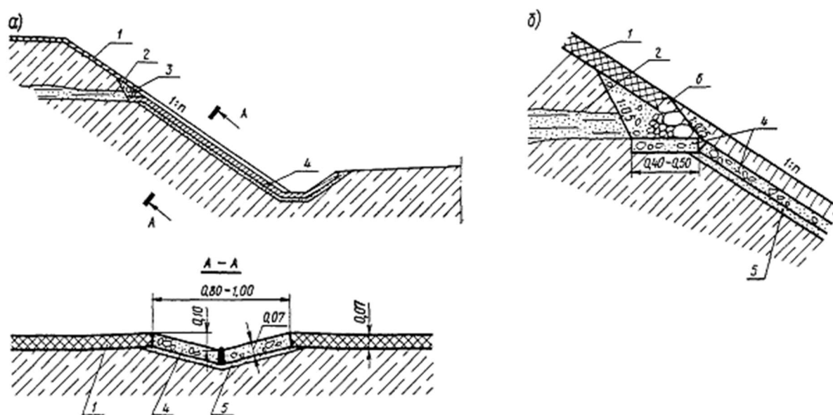
Рис. 4. Схема устройства открытого водоспуска:
