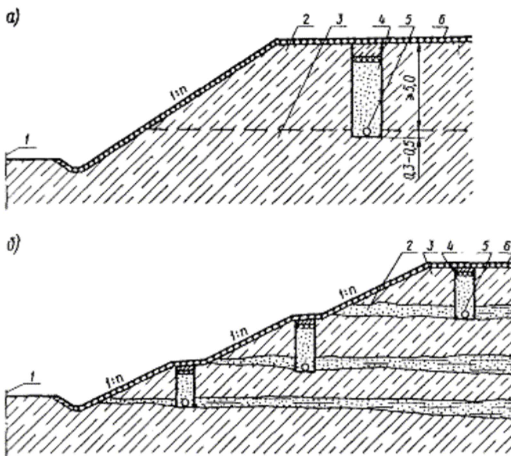
Рис. 5. Схема устройства ограждающего дренажа:
