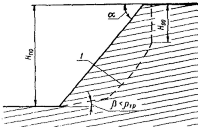
Рис. 5. Расчетная схема наклонного откоса при незначительном наклоне поверхностей ослабления:
