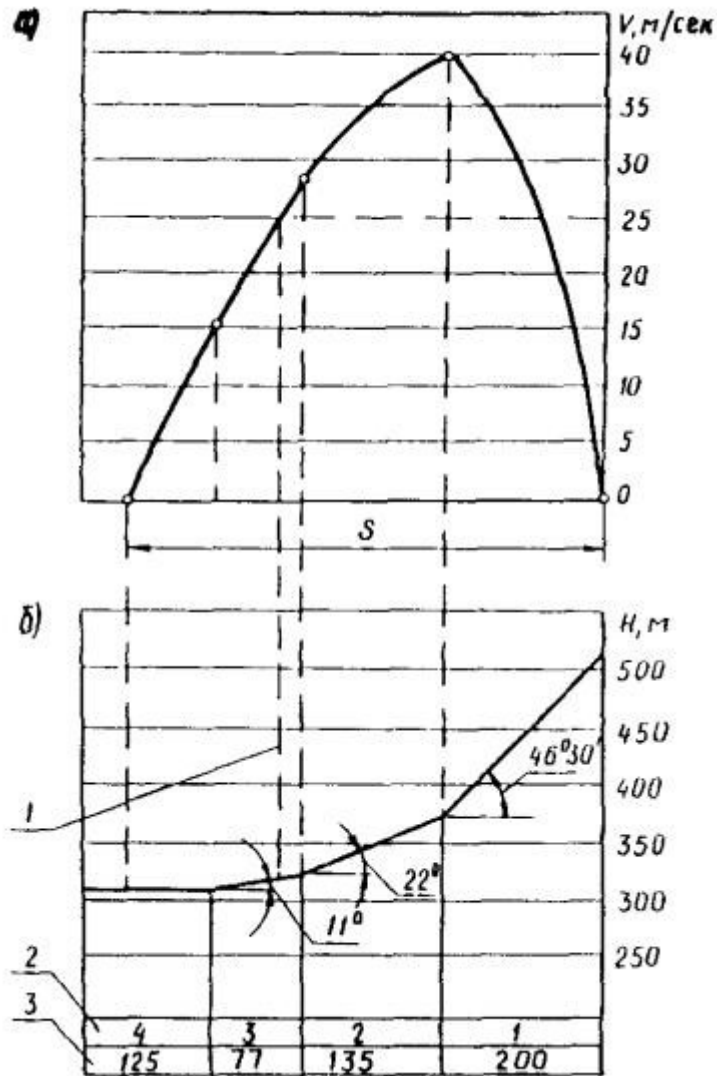
Рис. 5. Схема определения скоростей лавин:
