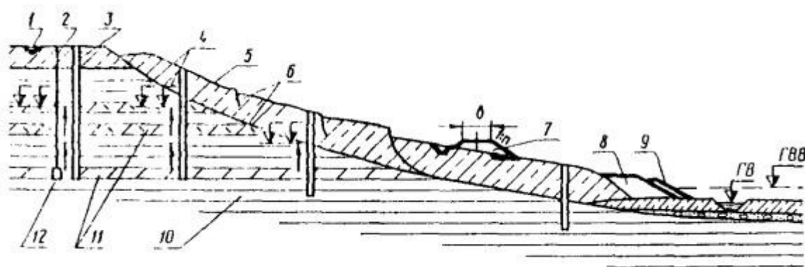
Рис. 24. Схема комплексного размещения противооползневых устройств:
