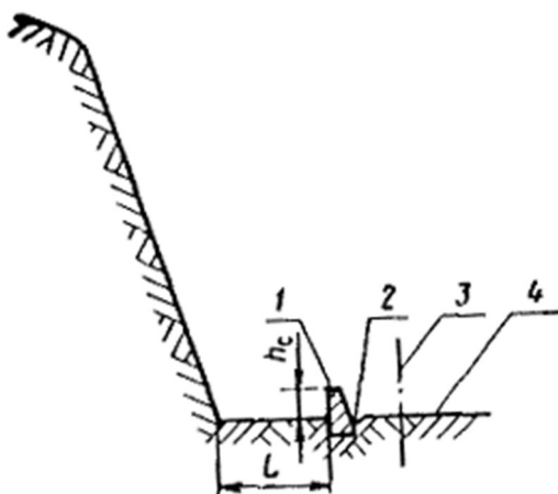
Рис. 34. Схема устройства путевой улавливающей полки с барьерной стенкой:
