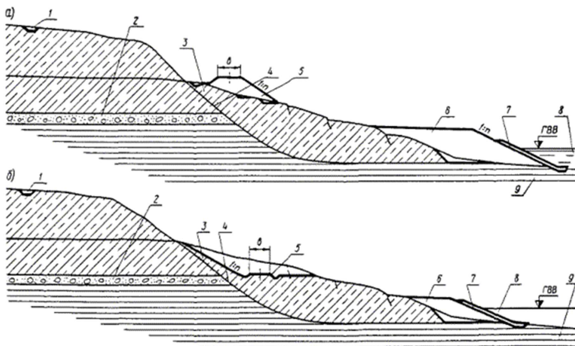
Рис. 15. Схема размещения земляного полотна в головной части оползневого массива и противооползневых устройств:
