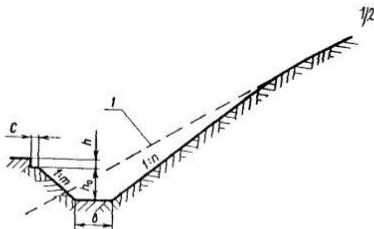
Рис. 5. Расчетная схема улавливающей траншеи:
