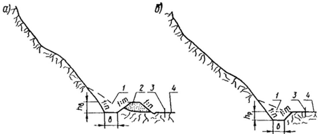
Рис. 36. Схема защиты полотна, размещенного у подошвы скально-обвального затяжного косогора:
