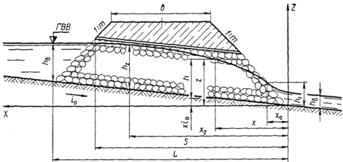
Рис. 2. Схема к гидравлическому расчету фильтрующих насыпей
