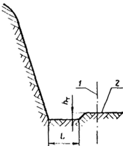
Рис. 33. Схема устройства путевой улавливающей траншеи:
