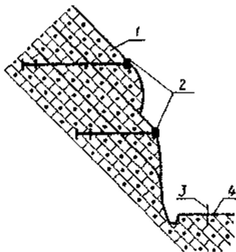
Рис. 32. Схема закрепления неустойчивых пластов породы:
