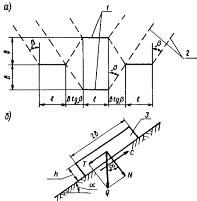
Рис. 1. Расчетные схемы удерживающих сооружений:
