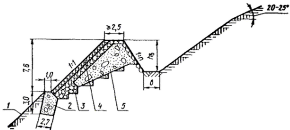
Рис. 39. Схема устройства улавливающего рва на косогоре крутизной от 20 до 25^\circ :
