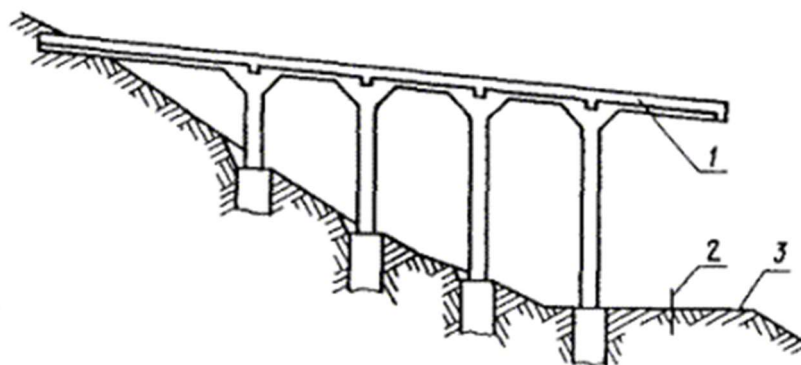
Рис. 47. Схема устройства железобетонного навеса над земляным полотном:
