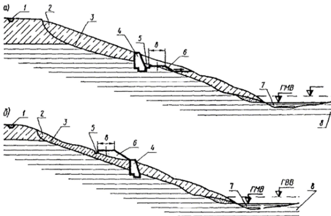
Рис. 17. Схема размещения земляного полотна с подпорными стенами на оползневом косогоре:
