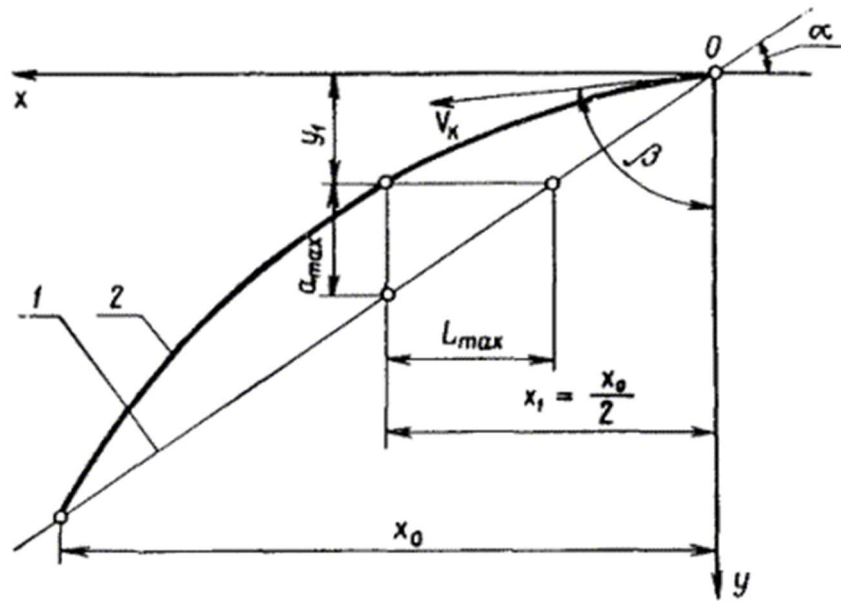
Рис. 2. Расчетная траектория движения камня после удара о наклонную плоскость:
