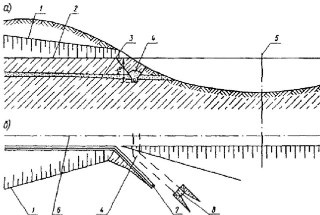
Рис. 13. Схема устройства дренажа-преградителя:
