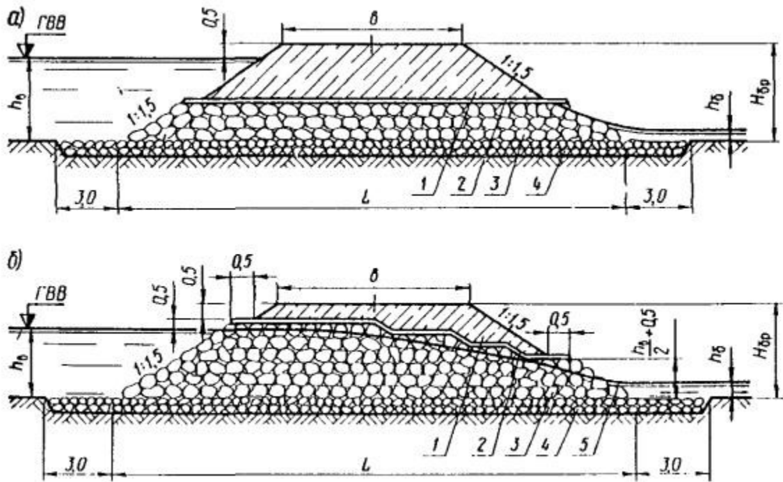
Рис. 1. Продольный разрез фильтрующих насыпей:
