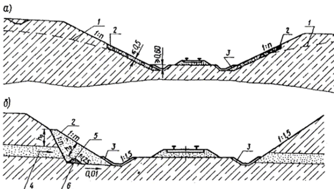
Рис. 3. Способы осушения грунта в откосах:
