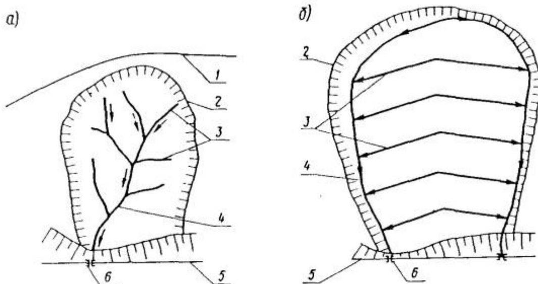
Рис. 21. Схемы размещения водоотводных канав в пределах оползневого массива:
