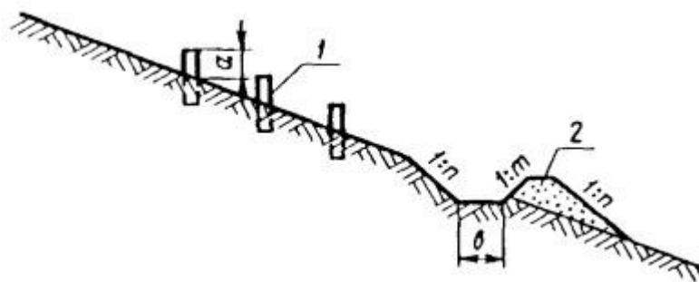
Рис. 43. Схема размещения надолб:
