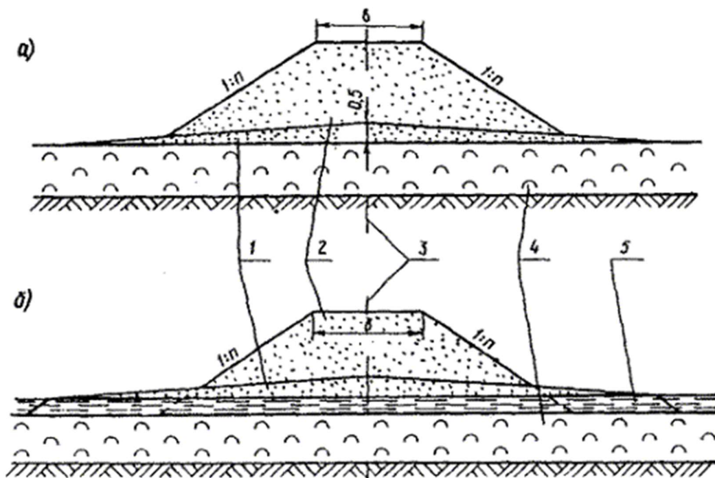
Рис. 49. Поперечные профили насыпи:
