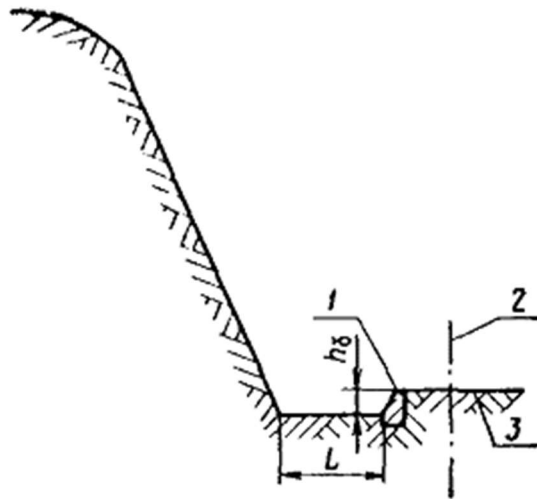
Рис. 35. Схема устройства путевой улавливающей полки с бордюрной стенкой:
