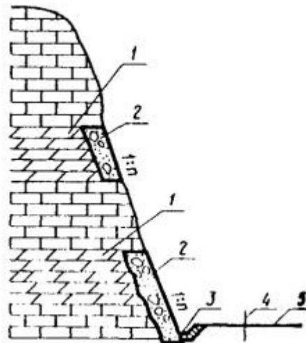
Рис. 28. Облицовочные стены:
