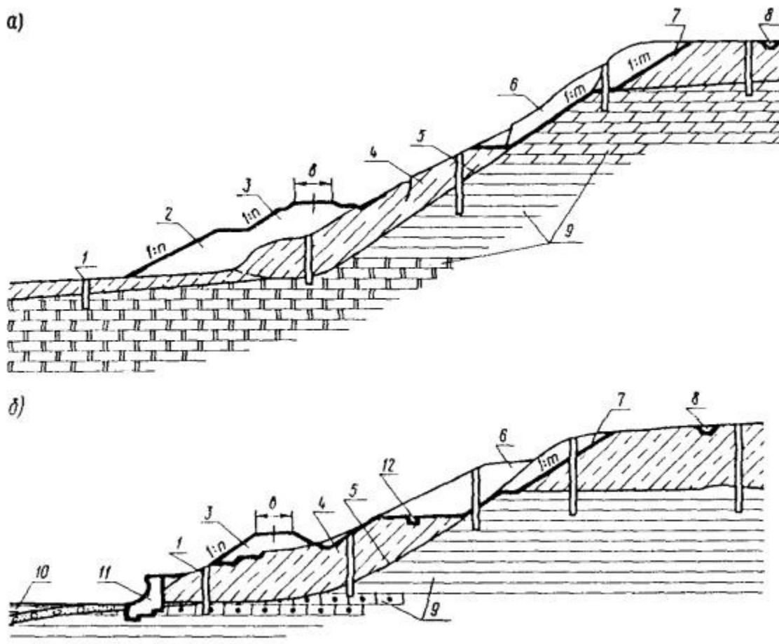
Рис. 18. Схема проектного решения по обеспечению устойчивости земляного полотна на оползневом косогоре:
