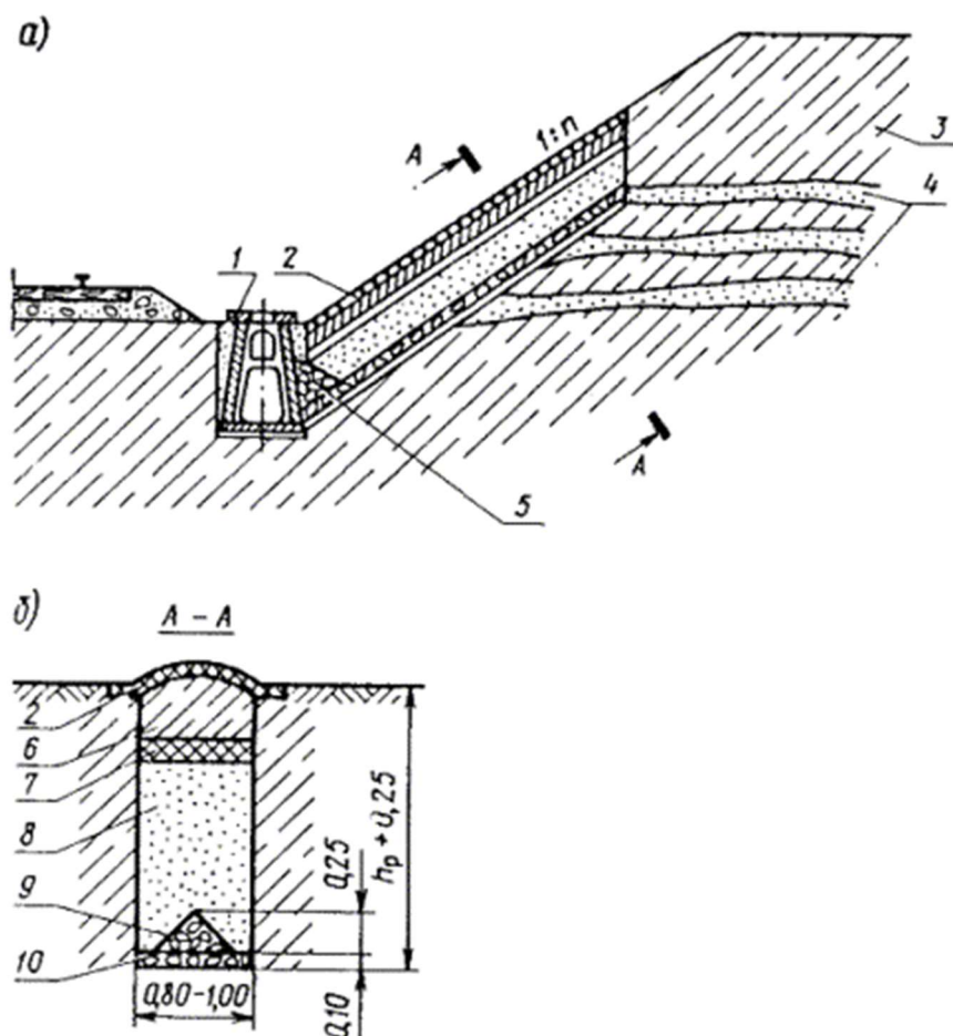
Рис. 2. Схема устройства откосного дренажа:
