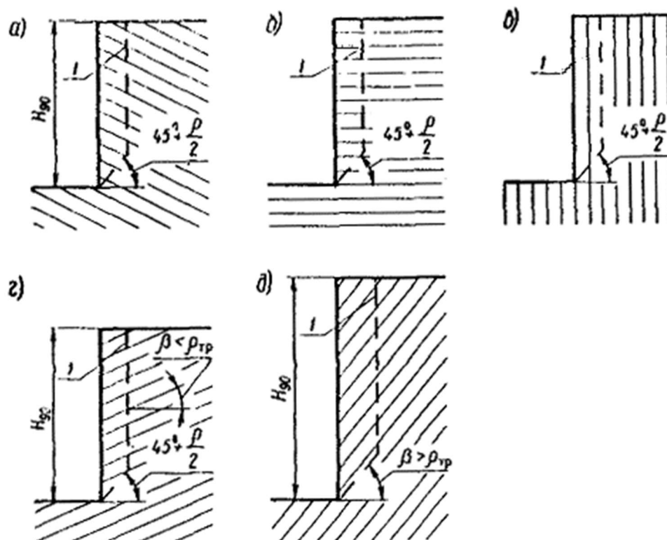
Рис. 1. Расчетные схемы вертикальных откосов:
