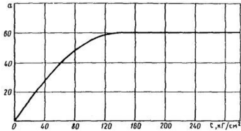
Рис. 2. График зависимости коэффициента \alpha от сцепления породы в образце
