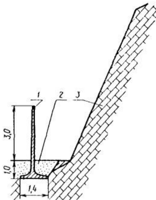
Рис. 41. Схема размещения барьерной улавливающей стены:
