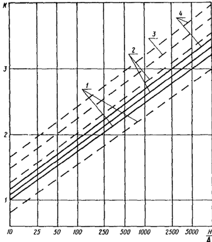
Рис. 1. График изменения коэффициента К:
