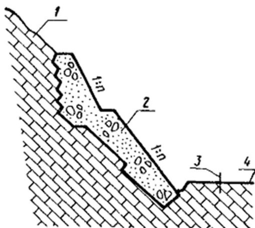
Рис. 29. Схема устройства контрфорса:
