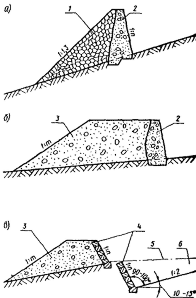
Рис. 45. Схема сооружений для задержания лавин:
