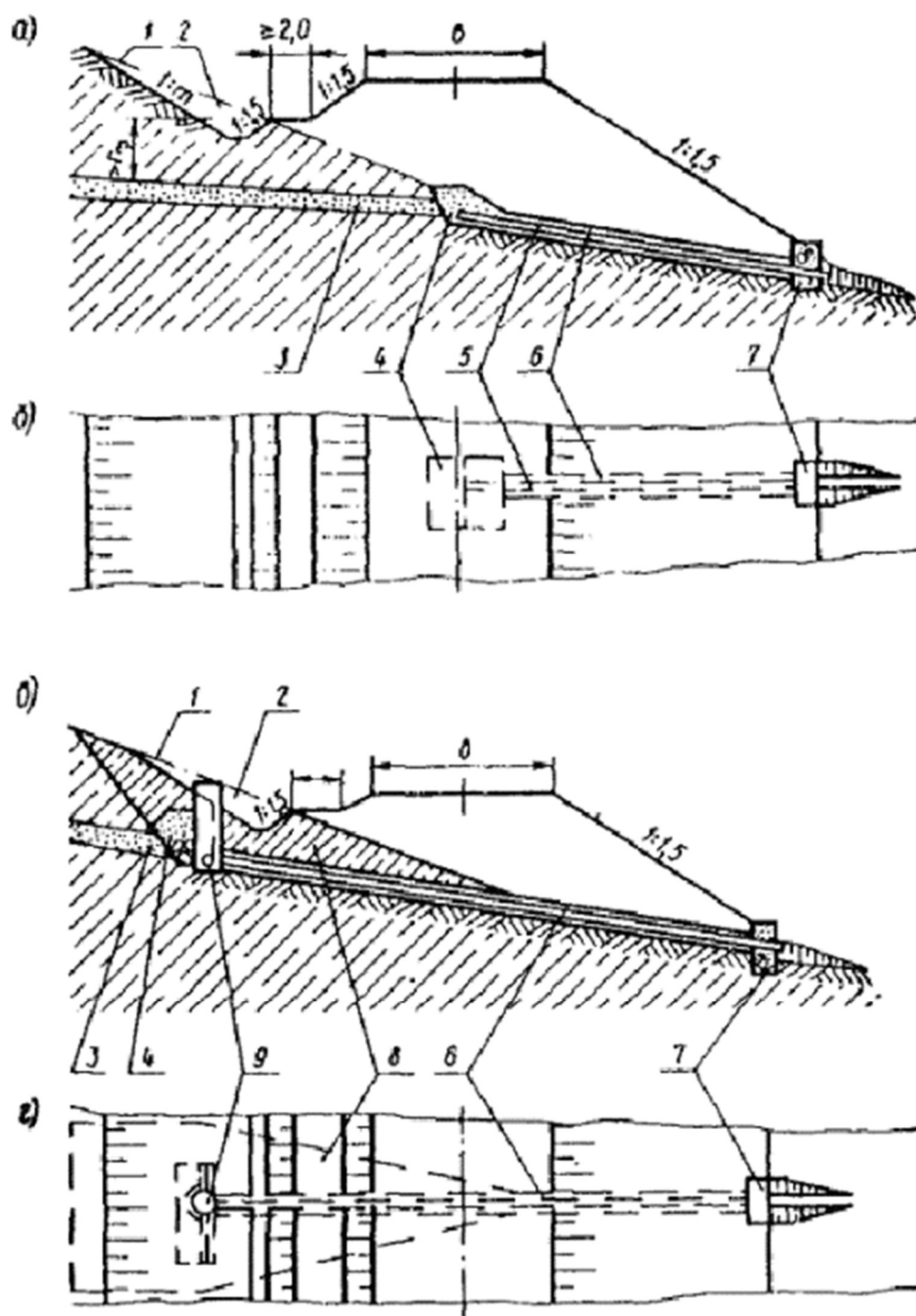
Рис. 12. Поперечные профили насыпей с каптирующими дренажными устройствами:
