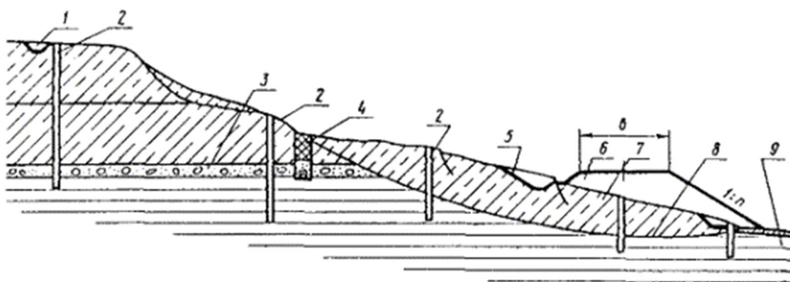
Рис. 22. Схема устройства земляного полотна на укрепляемом оползневом косогоре:
