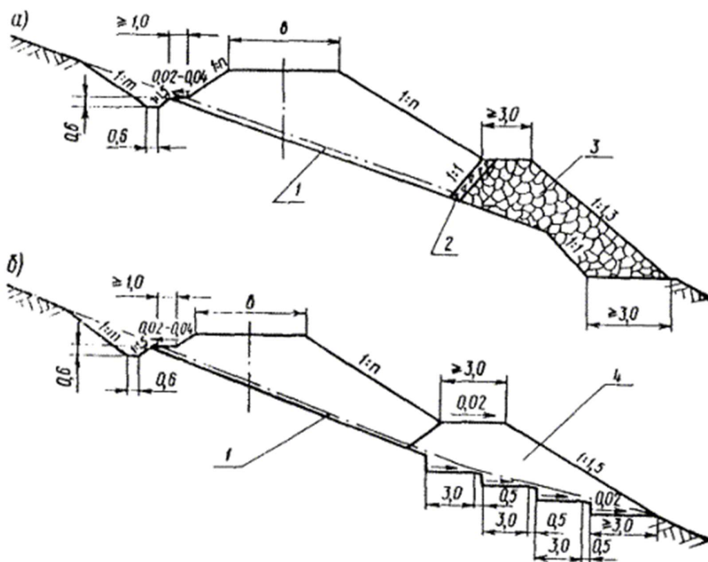
Рис. 8. Поперечные профили насыпей с упорными устройствами на крутых косогорах:
