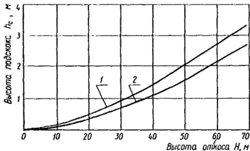
Рис. 2. График для определения высоты подскока камней:
