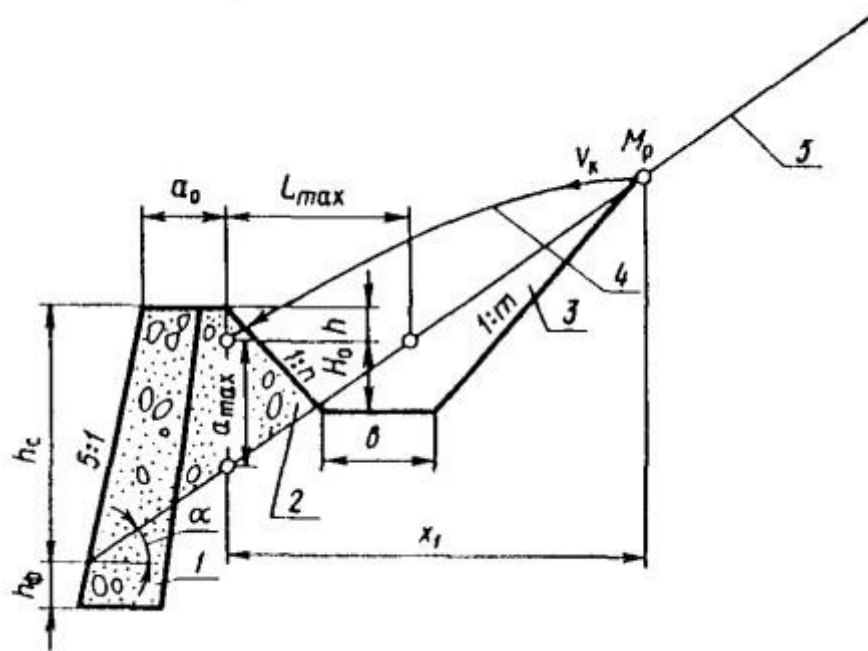
Рис. 3. Схема расчета ограждающего сооружения на перелет камня:
