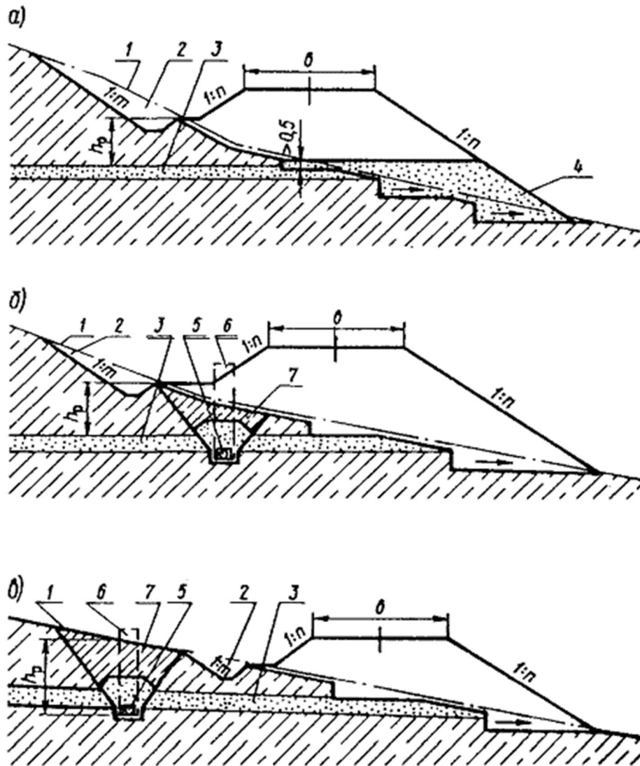
Рис. 11. Поперечные профили насыпей с дренажными устройствами в местах выхода грунтовых вод :
