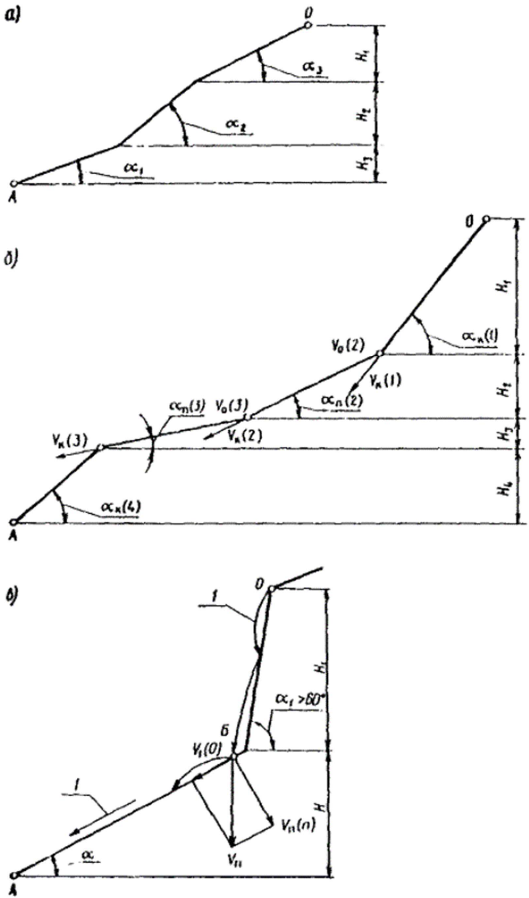
Рис. 1. Расчетные схемы склонов:
