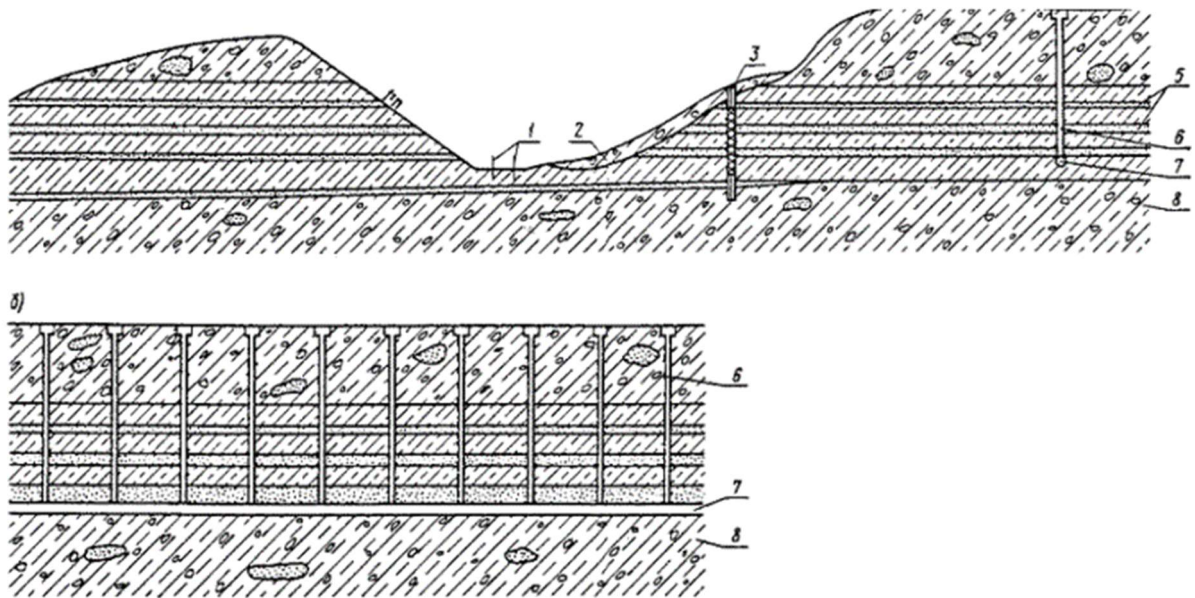
Рис. 6. Схема применения штольни для осушения откоса выемки:
