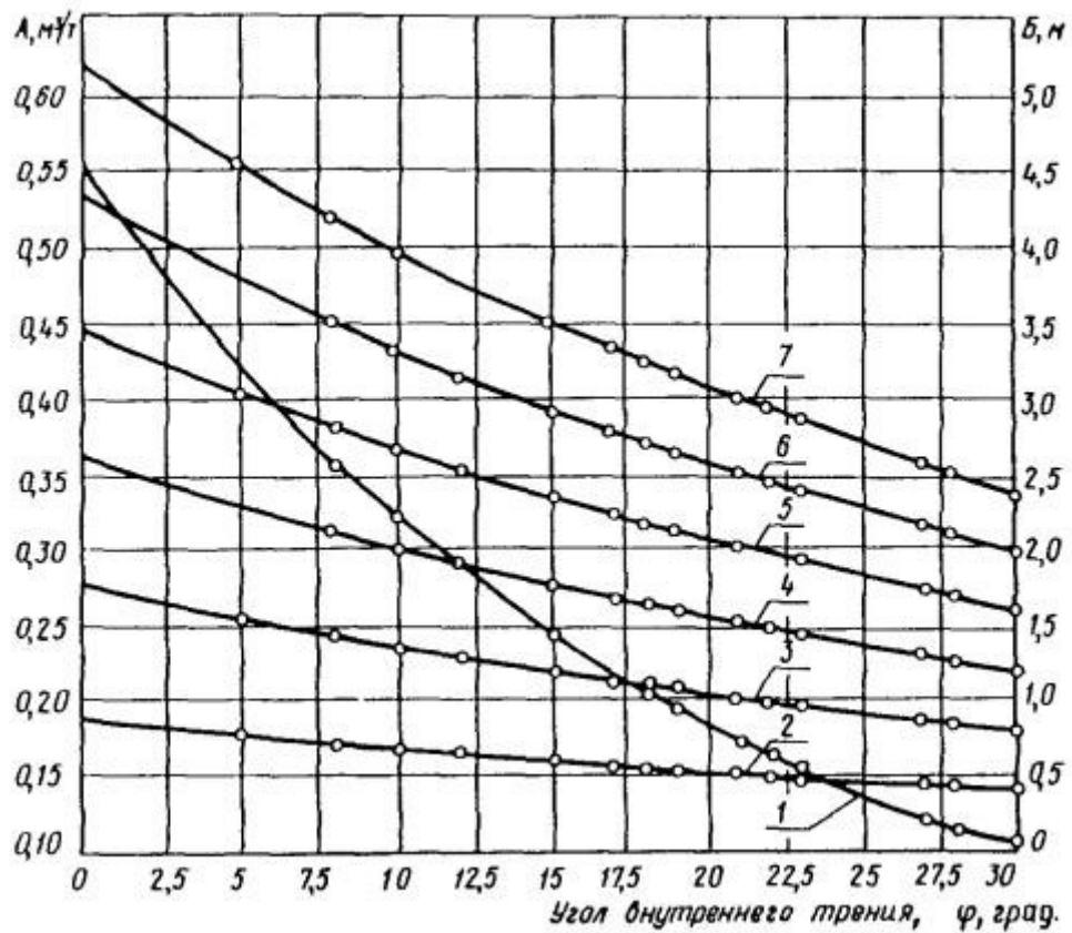
Рис. 2. Кривые зависимости параметров А и Б от прочностных характеристик грунта:
