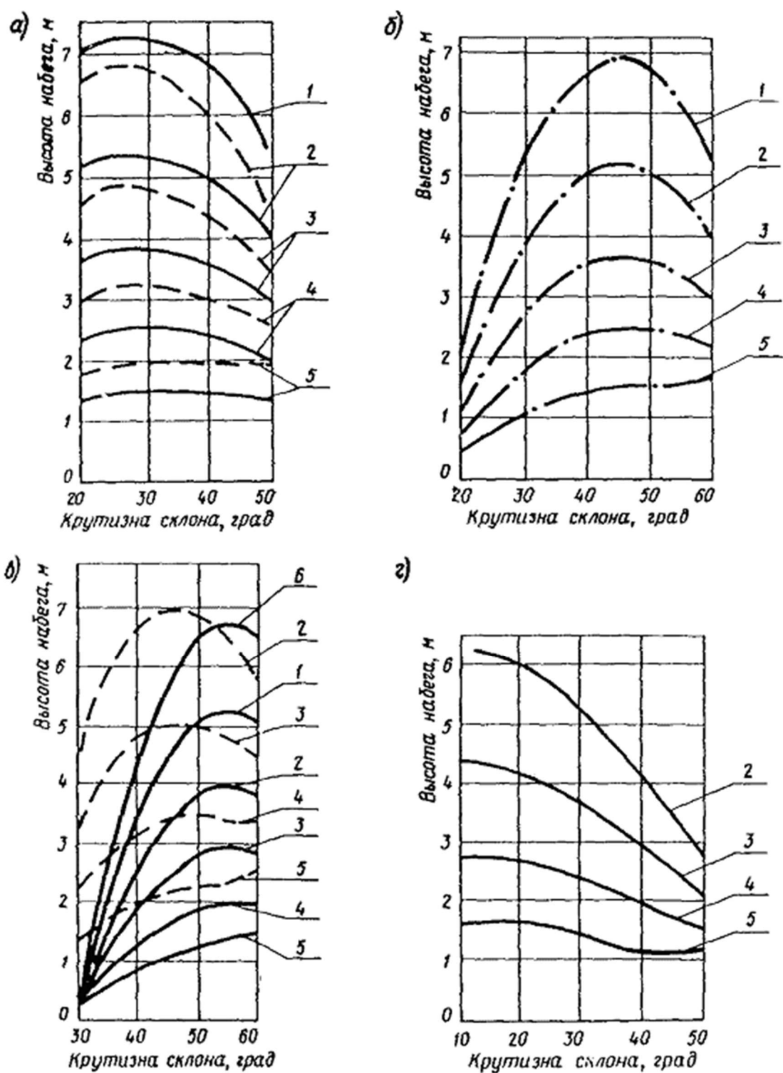
Рис. 4. Графики для определения высоты набега камней на откос:
