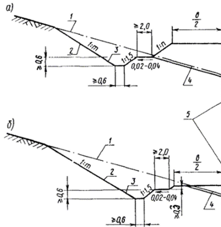
Рис. 10. Поперечные профили водоотводных канав, размещаемых в непосредственной близости от земляного полотна:
