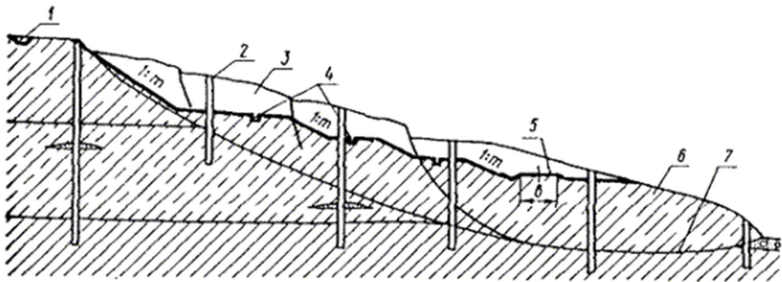
Рис. 19. Схема устройства земляного полотна с частичным удалением оползневого массива и террасированием откоса:
