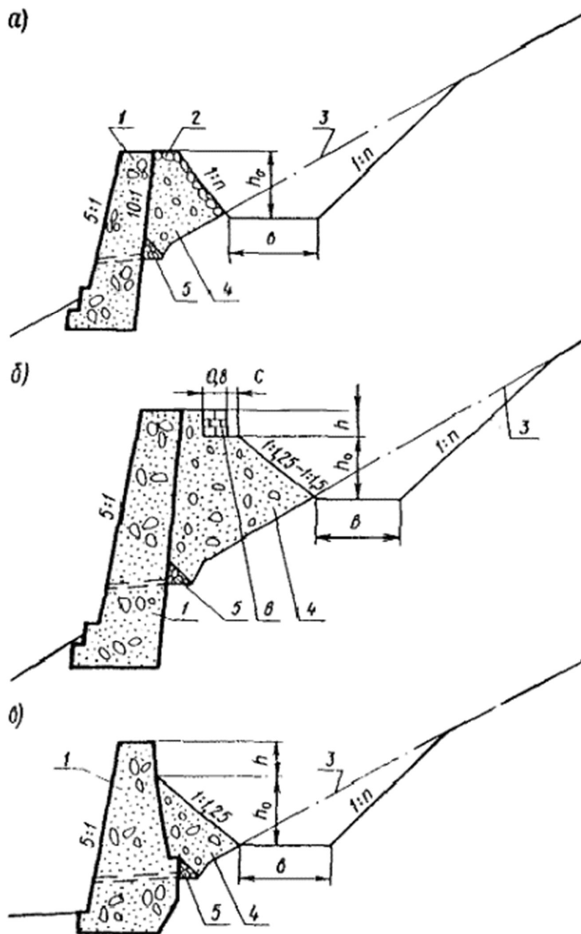
Рис. 42. Схемы улавливающих устройств:
