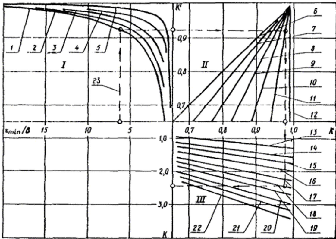
Рис. 3. Номограмма для определения значений коэффициента К для канав на закруглениях:
