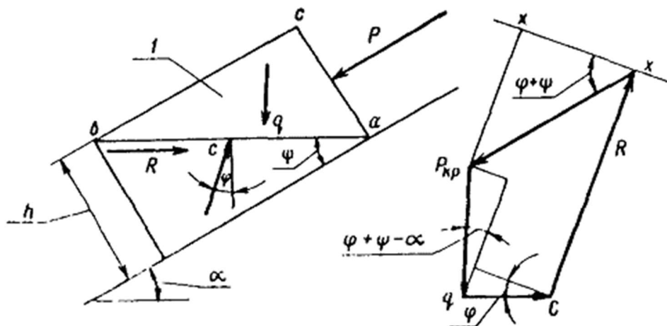
Рис. 2. Расчетная схема к определению критической нагрузки:
