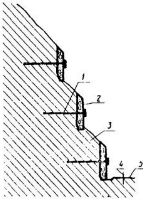
Рис. 27. Заанкеренные подпорные стены:
