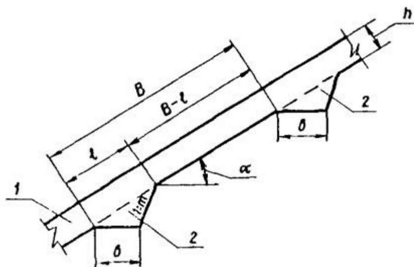
Рис. 4. Расчетная схема размещения террас:
