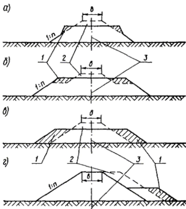
Рис. 48. Поперечные профили насыпей из дренирующих грунтов с размещением запасов грунта:
