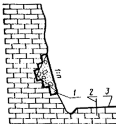
Рис. 30. Схема устройства пломбы:
