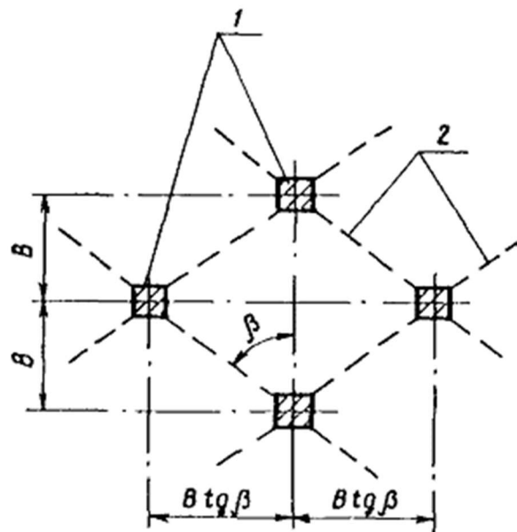
Рис. 3. Расчетная схема размещения свай в плане:
