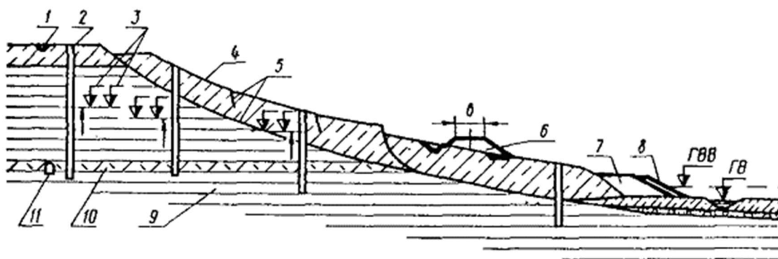
Рис. 23. Схема размещения противооползневых устройств:
