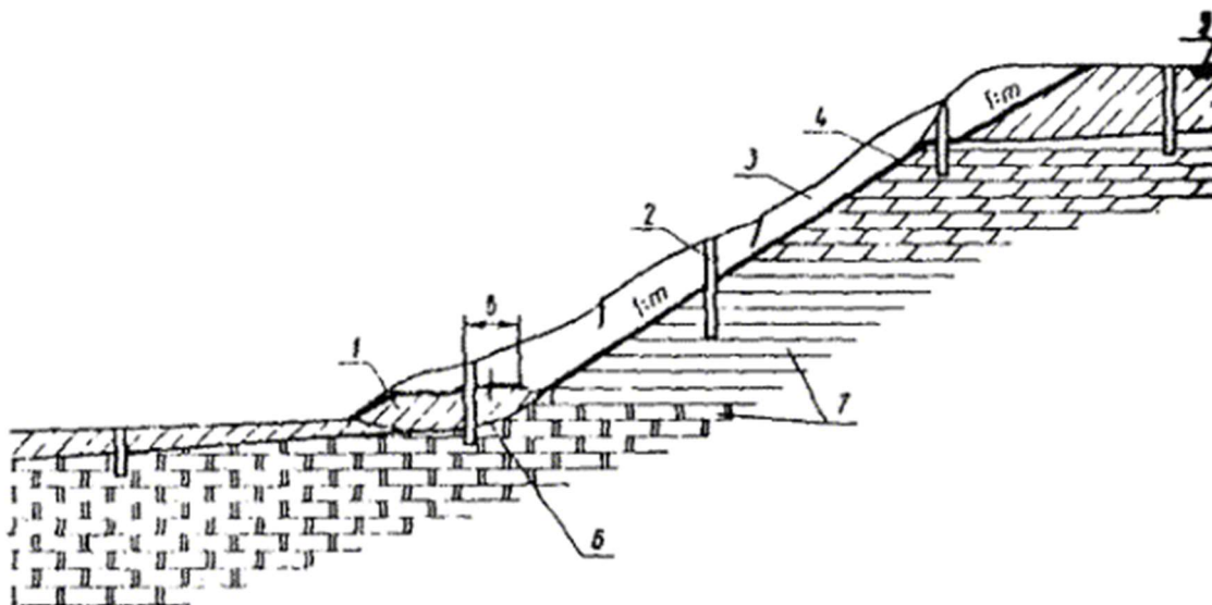
Рис. 20. Схема устройства земляного полотна с удалением оползневого массива:
