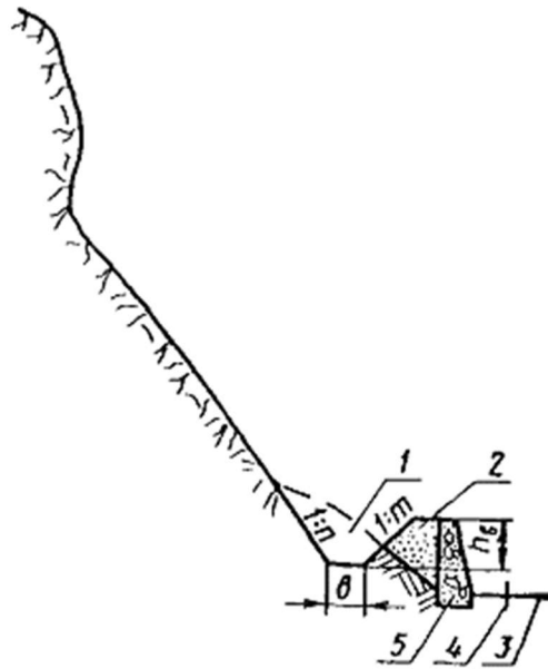
Рис. 40. Схема устройства улавливающей стены с застенной засыпкой:
