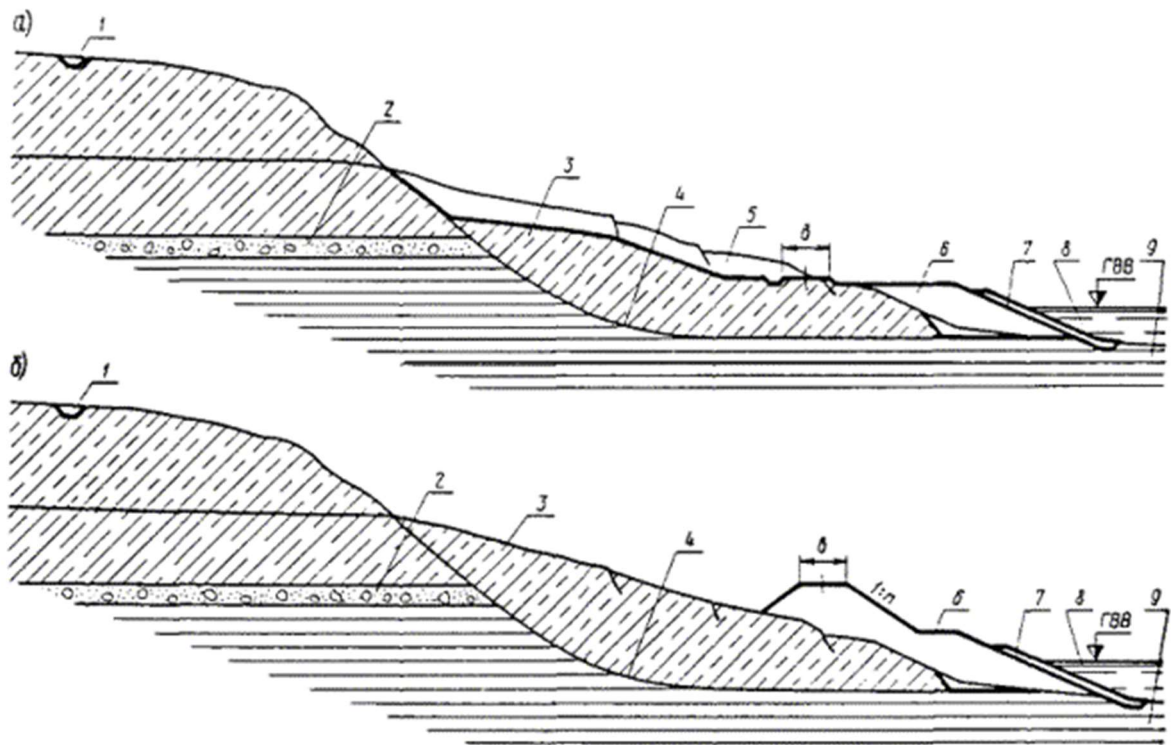
Рис. 14. Поперечный профиль насыпей с противодеформационными устройствами на оползневом косогоре:
