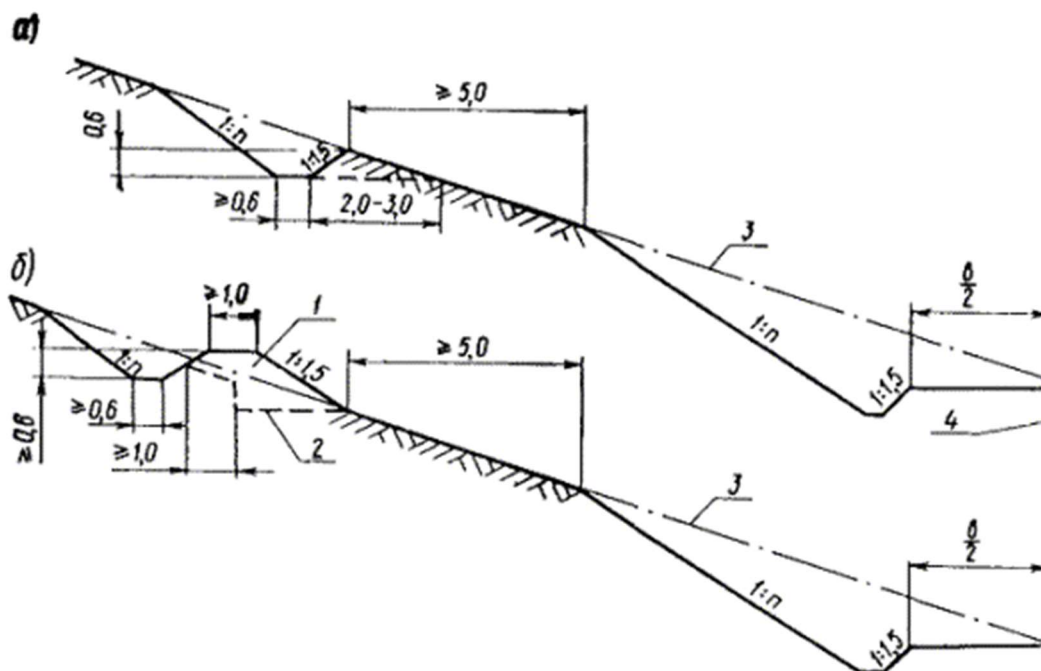
Рис. 9. Поперечные профили нагорных канав:
