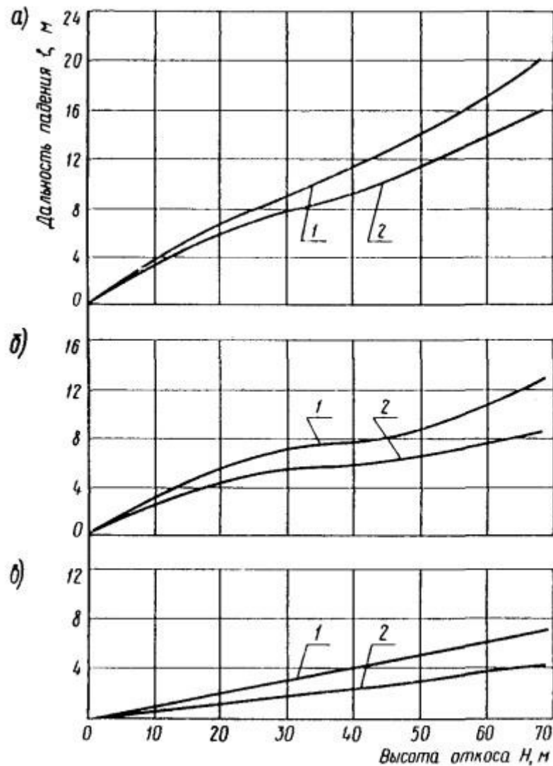
Рис. 1. Графики для определения дальности падения камней от подошвы откосов:
