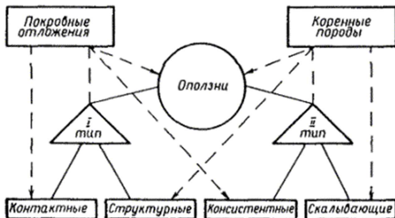
Рис. 1. Классификационная схема оползней
