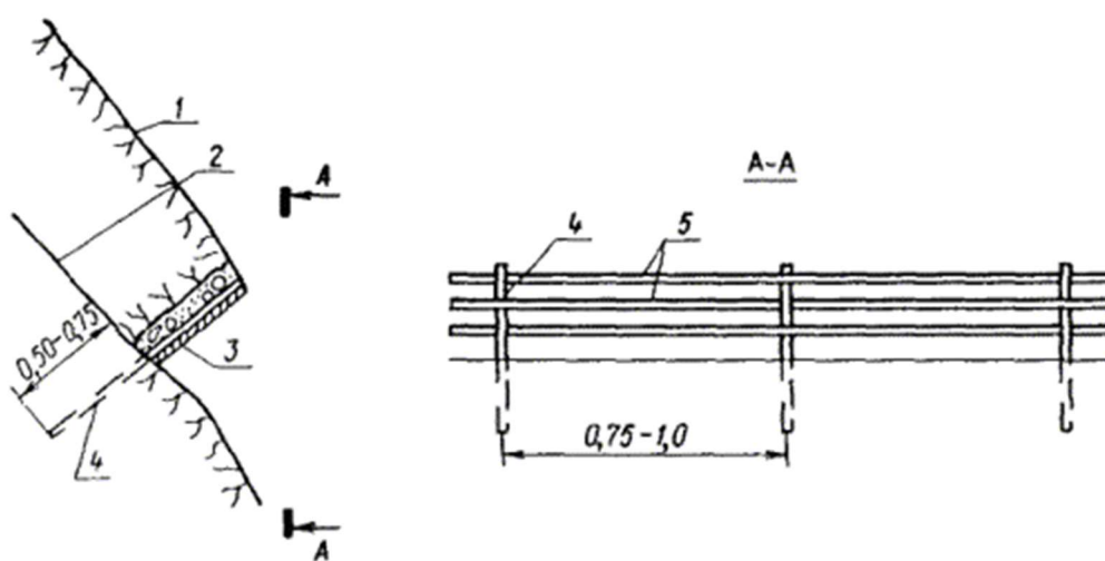
Рис. 31. Схема устройства опояски:
